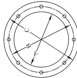
SAE FLANGE
